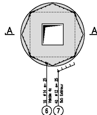
VUE EN PLAN 1:50 ARMATURE SECONDAIRE NIV. B-B+C-C
